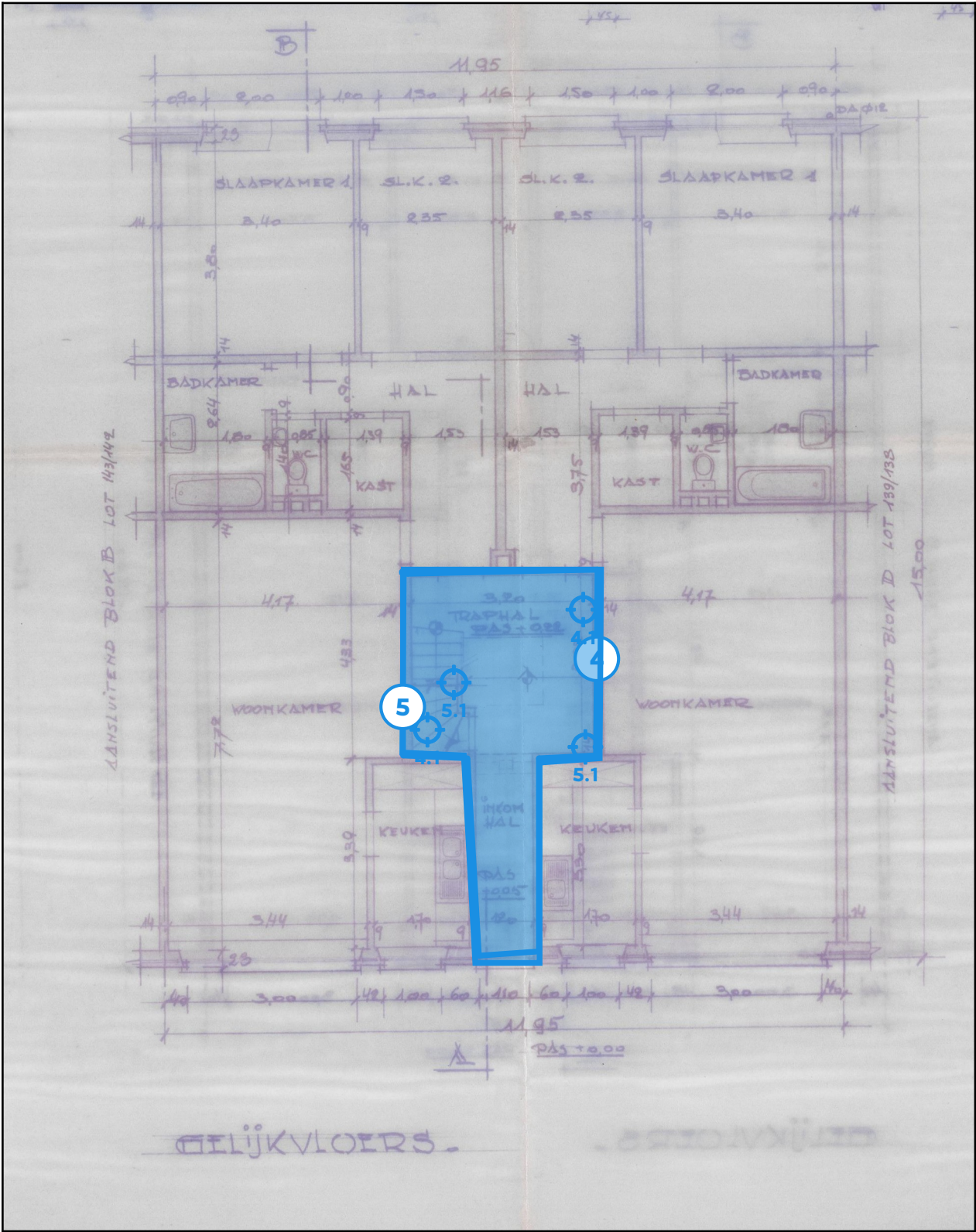
Legende van plan 1.4: 0 - Gelijkvloers
